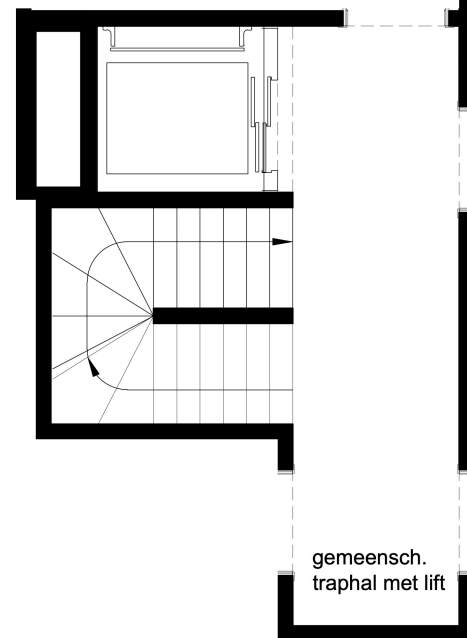
Grondplan
